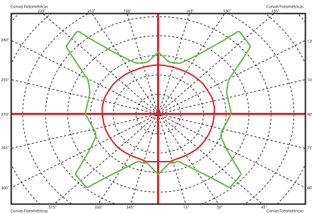
Curvas Fotométricas
